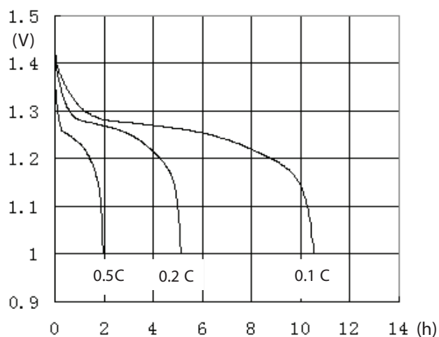
Vybíjecí charakteristika RAYLong 800 mAh 0,1-0,5C
