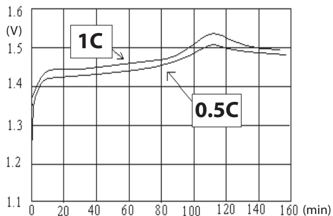
Nabíjecí charakteristika RAYLong 800 mAh
