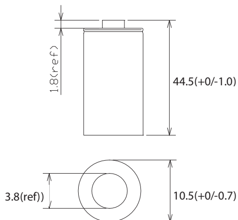
Rozměrový výkres
