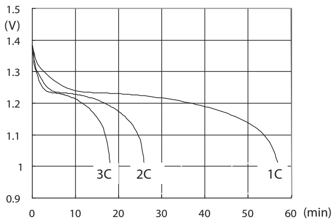
Vybíjecí charakteristika RAYLong 800 mAh 1-3C
